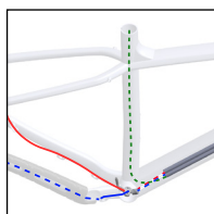
Cablagem — espigão telescópico, sem desviador dianteiro
