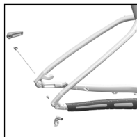
Desviador traseiro e bloqueio de roda
