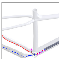
Cablagem — desviador dianteiro, sem espigão telescópico
